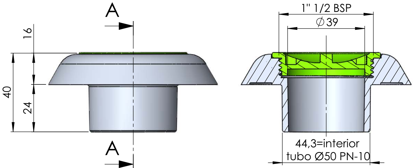
SECCIÓN A-A
