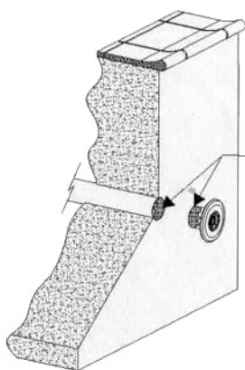
Установка на бассейн с трубой из ПВХ Ø 63 мм
