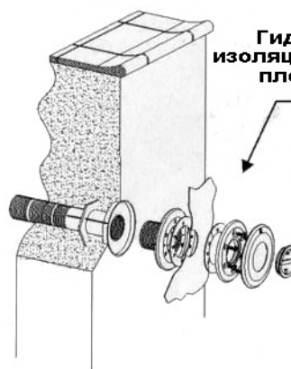
Установка на бассейн с нарезной трубкой в стенке бассейна (код 15663, 15664 и 15665) и гидроизоляционной пленкой
