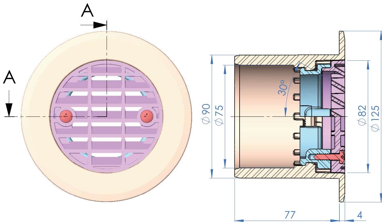
SECCIÓN A-A
