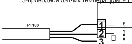
3-проводной датчик температуры PT100
