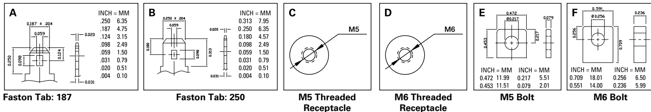
Faston Tab: 187
